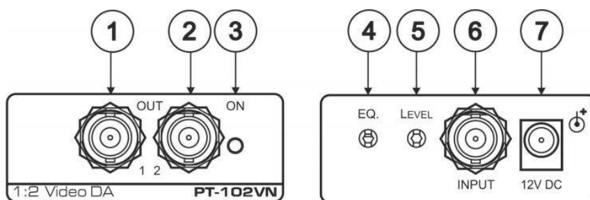
図 1 : PT-102VN 1:2 コンポジットビデオ分配器
