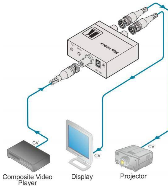
図 2 : PT-102VN 1:2 コンポジットビデオ分配器の接続
